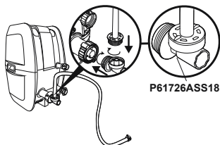
Schnellventil zum Aufblasen und Entleeren
